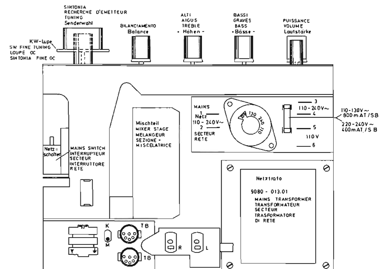
Buchsen- und Anschlußseite SOCKET AND CONNECTION SIDE COTE DE PRISES ET CONNEXIONS LATO PRESE E COLLEGAMENTO
