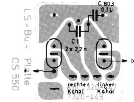
Lautsprecher-Buchsenplatte, Lötseite SPEAKER SOCKET PLATE, SOLDER SIDE PLAQUE PRISES HP, COTE DES SOUDURES PIASTRE PRESE ALTOPARLANTI, LATO SALDATURE
