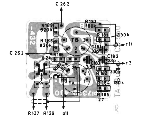
TA-TB-Buchsenplatte, Lötseite PU-TR-SOCKET PLATE, SOLDER SIDE PLAQUE PRISES PU/MAGNETO, COTE DES SOUDURES PIASTRA PRESE FONOREGISTRATORE, LATO SALDATURE
