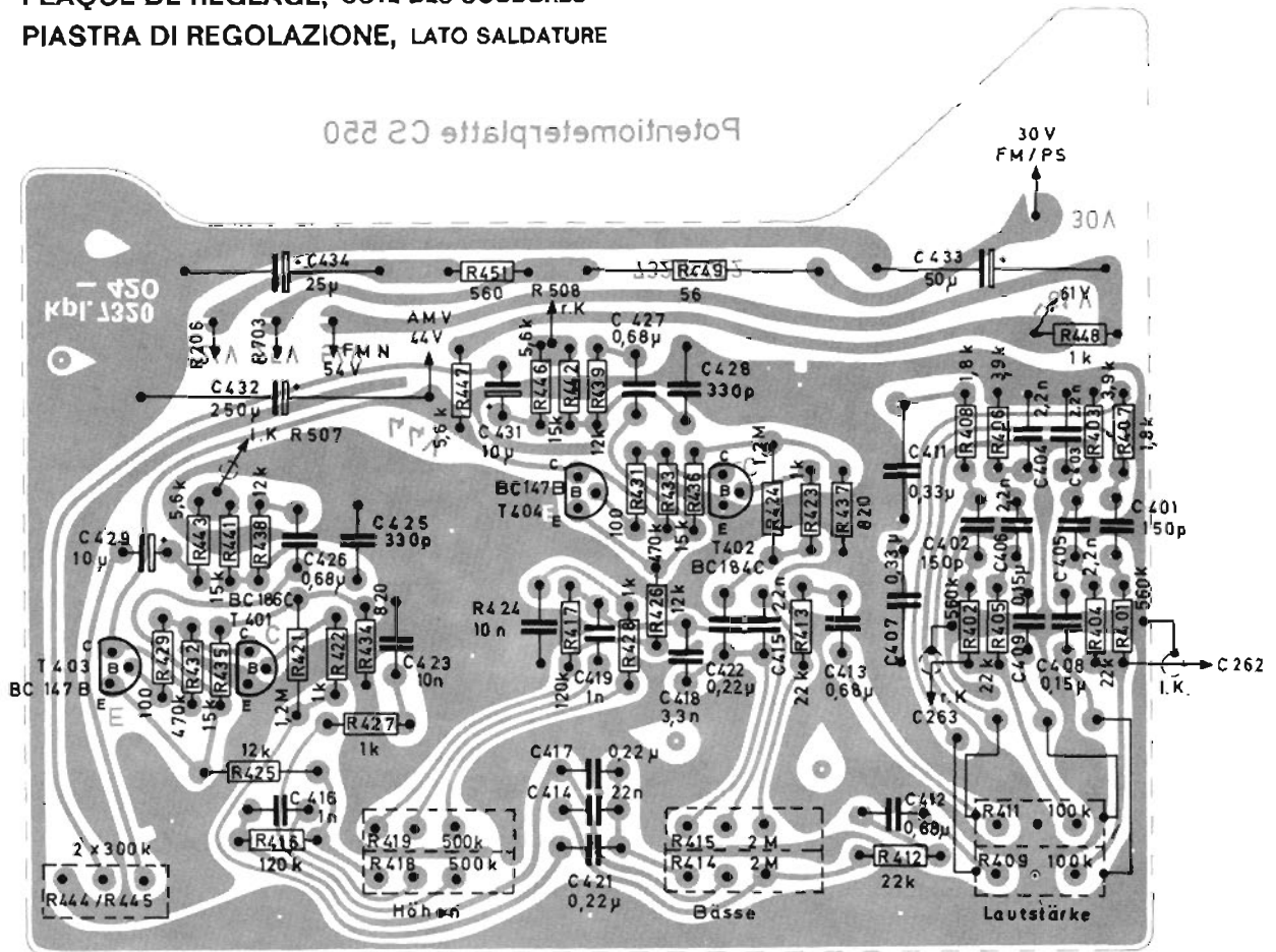
Potentiometerplatte, Bestückungsseite POTENTIOMETER BOARD, COMPONENT SIDE PLAQUE DE REGLAGE, VUE DU COTE DES COMPOSANTS PIASTRA DI REGOLAZIONE, LATO COMPONENTI
