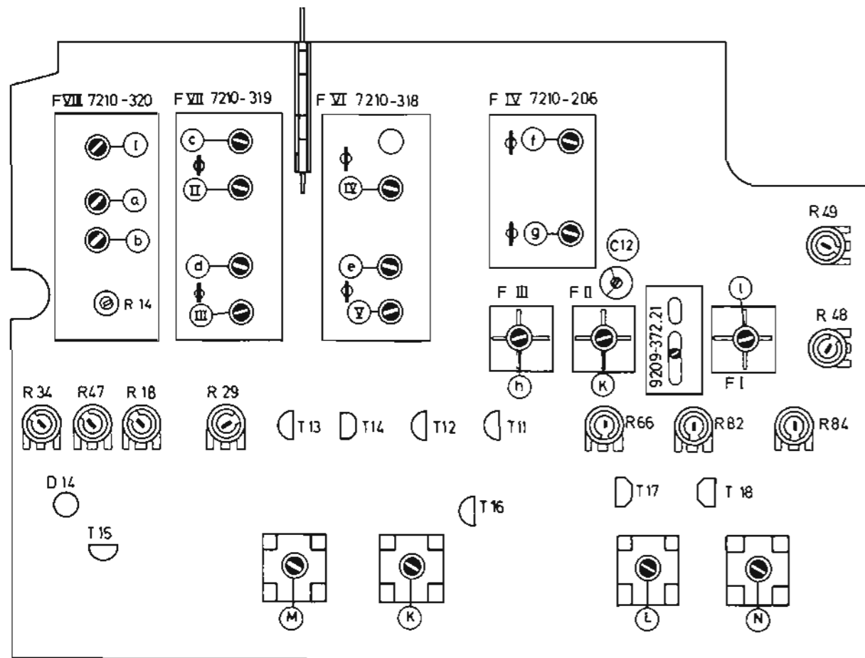
Abgleich-Lageplan, AM-FM, ZF und Decoder ALIGNMENT SCHEME, AM-FM, IF AND DECODER PLAN DE REGLAGE, AM-FM, FI ET DECODEUR PIANO DI TARATURA, AF-FM, FI ED DECODER
